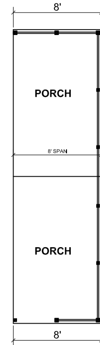
OPTIONAL PORCH
